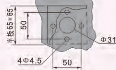
柜外手柄座安装尺寸
