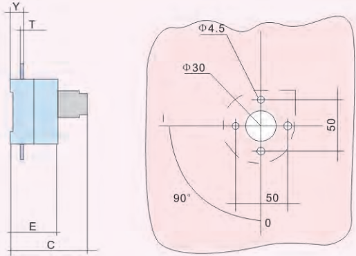
柜外手柄座安装尺寸
