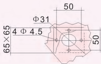
柜外手柄座安装尺寸
