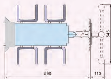
柜外手柄安装尺寸
