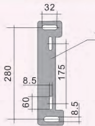
柜外操作安装底板
