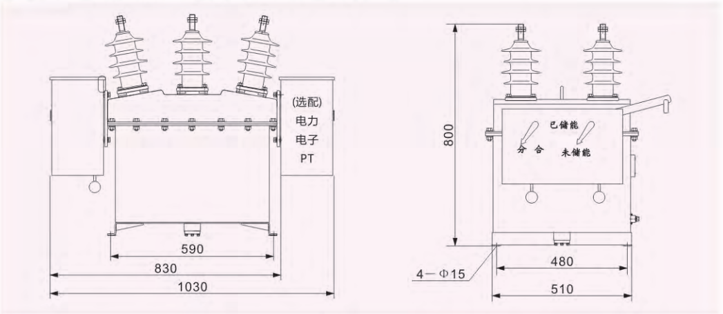
2、ZW8-12G(带隔离)真空断路器外形及安装尺寸(单位：mm)
